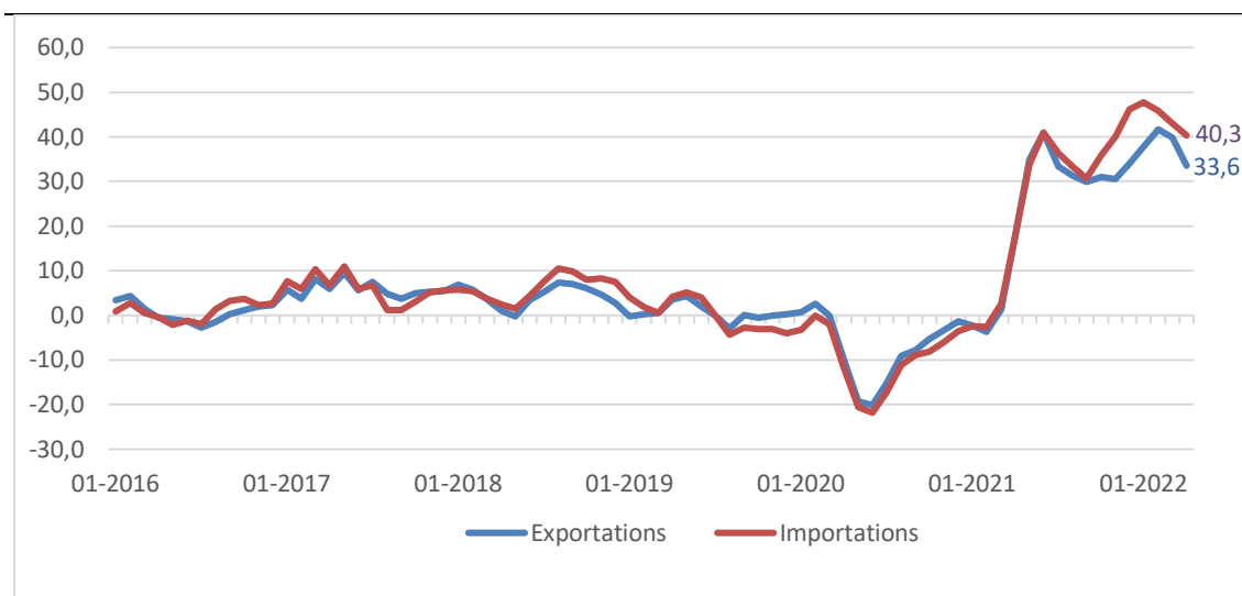
GRAPHIQUE 1 – ÉVOLUTION DES IMPORTATIONS ET EXPORTATIONS DE BIENS 1
